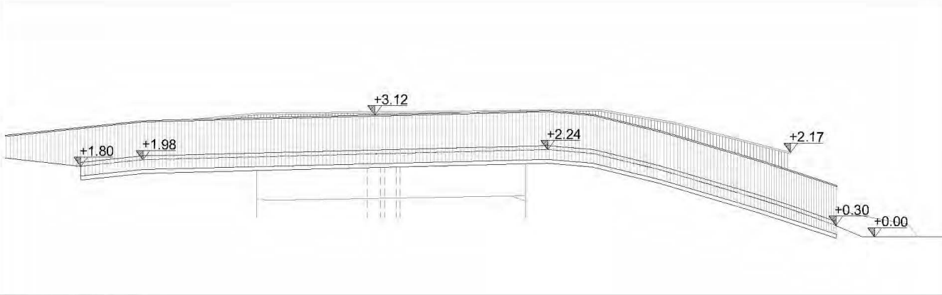
PROSPETTO SUD SC. 1:100
