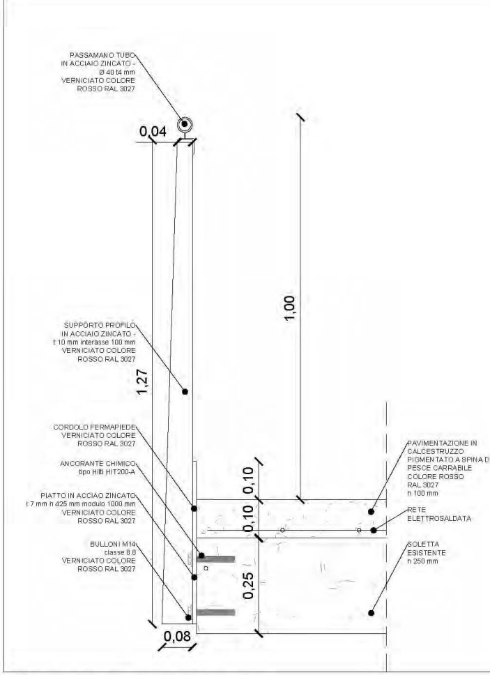
SEZIONE TIPOLOGICA PARAPETTO SC. 1:10
