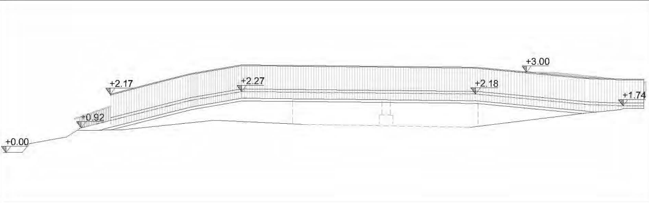
PROSPETTO NORD SC. 1:100
