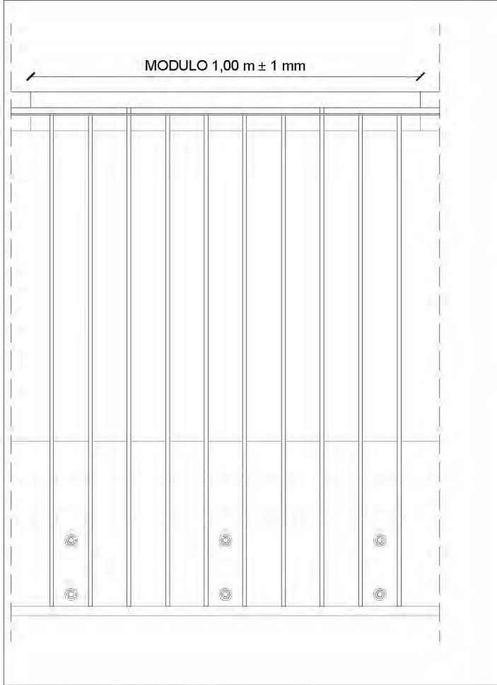
PROSPETTO TIPOLOGICO PARAPETTO SC. 1:10
