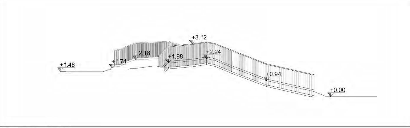
PROSPETTO OVEST SC. 1:100
